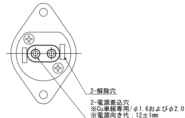
[ソケット-配線側]
