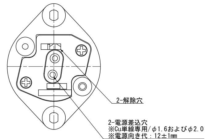
[ソケット-配線側]
